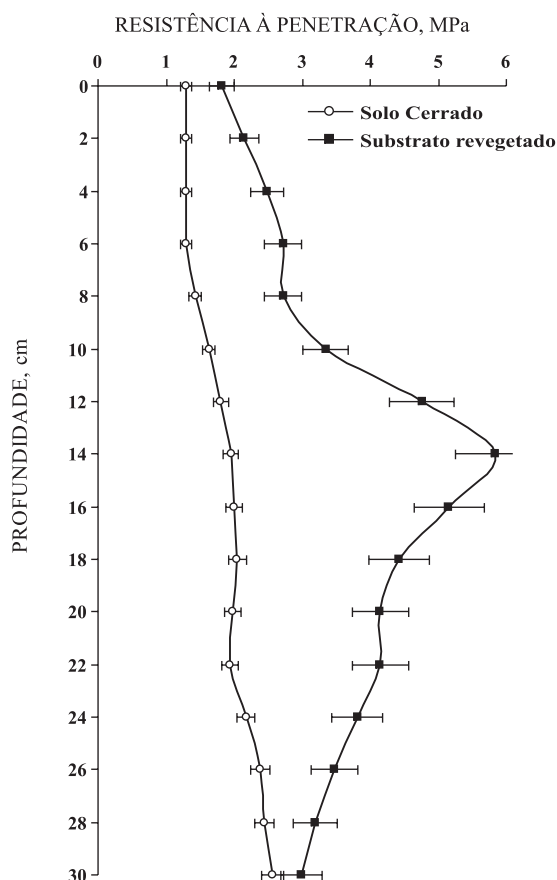
Figura 1. Resistência mecânica à penetração para o substrato revegetado e para o solo sob Cerrado nativo.
