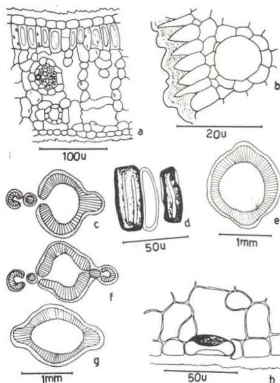
Fig. 1 — Lorostemon coelhoi — a) corte transversal da lâmina foliar, onde se vêem um feixe vascular envolvido por uma bainha fisiológica, um canal secretor e grandes lacunas; b) caule: estrutura primária mostrando a epiderme e um canal; c) sistema vascular do nó foliar na altura da metade de seu comprimento, onde se vêem os cordões vasculares do rastro foliar; d) células do parênquima paliçádico dissociadas; e-g) sistema vascular da base do nó foliar; f) sistema vascular da porção mais alta do nó foliar, mostrando dois cordões vasculares do rastro foliar; h) estômatos em secção transversal.
