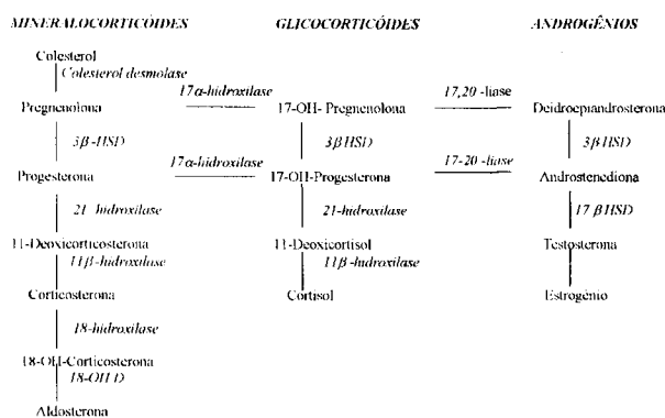
Figura 1. Principais etapas da esteroidogênese adrenal (3 \beta -HSD = 3beta-hidroxisteróide desidrogenase; 18-OHD = 18-hidroxidesidrogenase)
