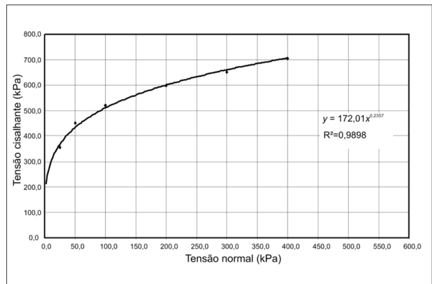
Figura 2 - Envoltória de resistência da Cava Crista.
