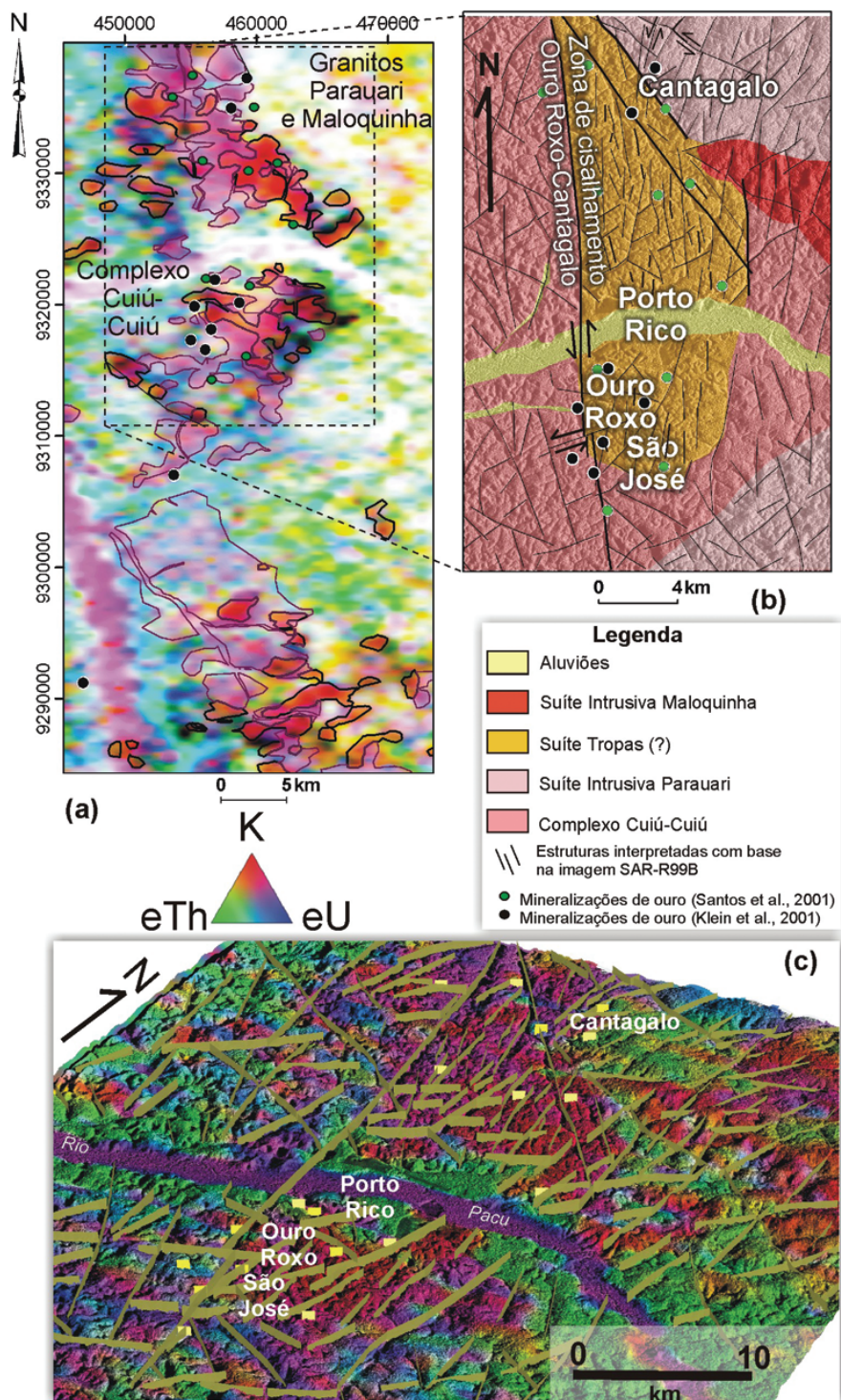
Figura 3 – Resultados gerados para a área Ouro Roxo-Cantagalo: (a) imagem de K, eTh e eU (RGB) com interpretação de unidades litogeofísicas de médio a alto K; (b) interpretação integrada de dados gamaespectrométricos e do SAR-R99B visando o reconhecimento de estruturas e unidades litogeofísicas; e (c) destaque da unidade litogeofísica de alto K normalizado caracterizada por proeminente trend estrutural NNE-SSW, assim como pela zona de cisalhamento Ouro Roxo-Cantagalo, de direção aproximada N-S. As mineralizações estão indicadas pelos polígonos em amarelo.
