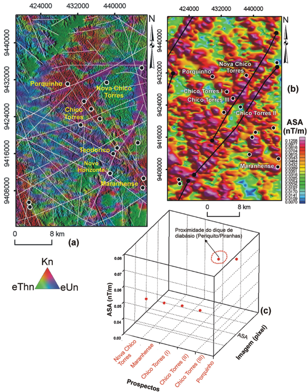
Figura 7 – Integração da imagem SAR-R99B ( L_{HH} ) com a da composição ternária RGB de Kn, eThn e eUn (a), incluindo os principais alinhamentos de drenagem. Imagem da amplitude do sinal analítico (ASA) integrada com ocorrências auríferas é mostrada em (b). Um gráfico tridimensional contendo as respostas extraídas de pixels da imagem da ASA referentes aos principais prospectos da região é apresentado em (c). Notar que altas amplitudes do sinal analítico estão associadas a alguns prospectos, e devem-se às respostas de diques máficos, os quais ainda não estão claramente definidos quanto a uma possível relação com as mineralizações auríferas.
