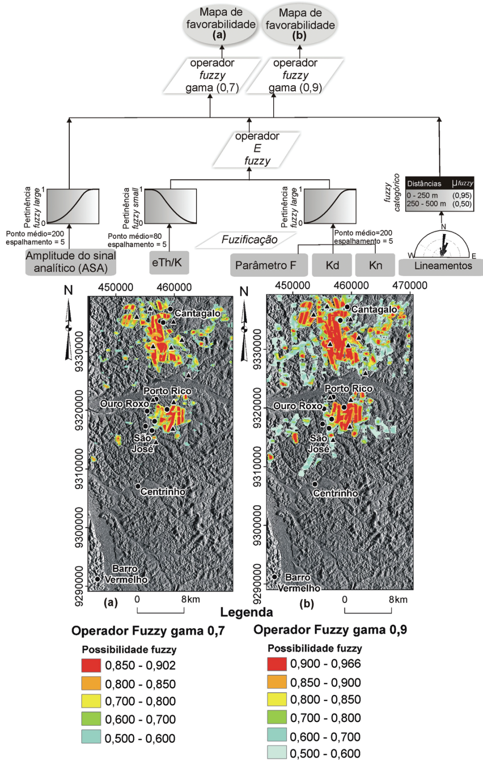
Figura 5 – Aplicação da lógica fuzzy na região Ouro Roxo-Cantagalo. Os mapas de favorabilidade aurífera foram produzidos pelos seguintes operadores fuzzy : (a) fuzzy gama (0,7); (b) fuzzy gama (0,9). Triângulos pretos compreendem as ocorrências de ouro identificadas em Santos et al. (2001) e círculo pretos aquelas indicadas em Klein et al. (2001).
