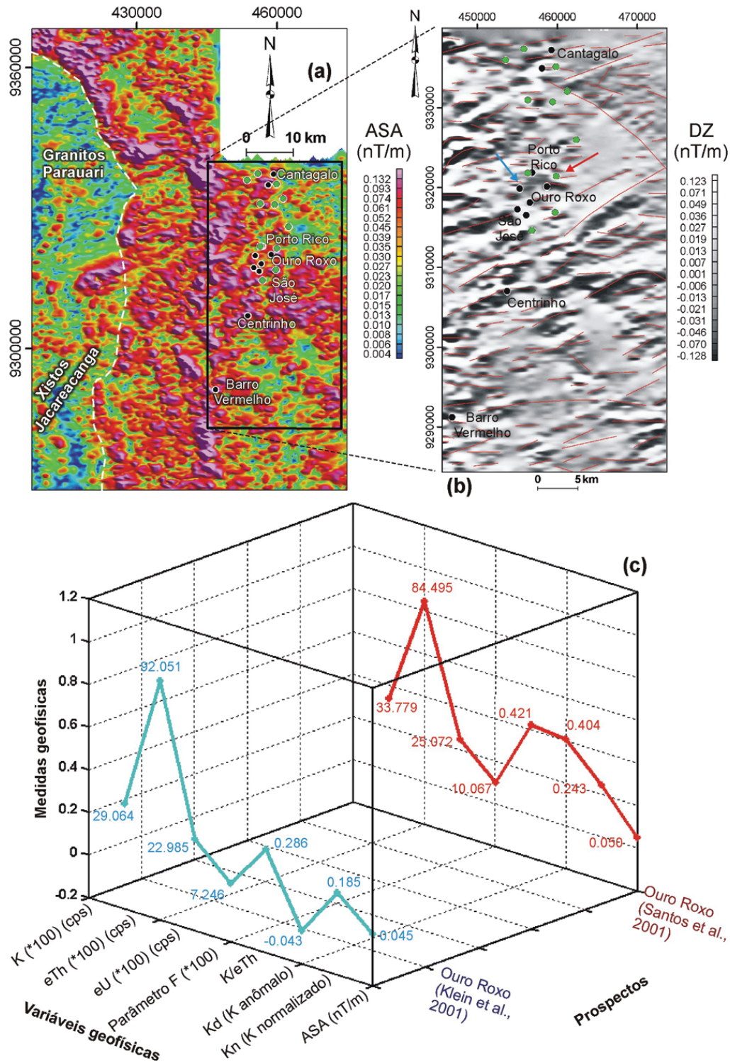
Figura 4 – Imagens magnetométricas da região Ouro Roxo-Cantagalo: (a) a ASA e a interpretação, em linha tracejada branca, de Silva (2003) e Silva et al. (2007) equivalente ao possível registro da subducção de crosta oceânica e formação do arco Cuiú-Cuiú; (b) imagem da primeira derivada vertical do campo magnético anômalo e interpretação de feições magnéticas. Seta azul indica a localização do prospecto Ouro Roxo por Klein et al. (2001), enquanto a seta vermelha refere-se ao mesmo prospecto de acordo com Santos et al. (2001). As características gamaespectrométricas e magnetométricas pontuais destas duas bases georreferenciadas do prospecto Ouro Roxo são mostradas em (c), podendo-se verificar grandes diferenças, principalmente das medidas gamaespectrométricas que realçam o K.
