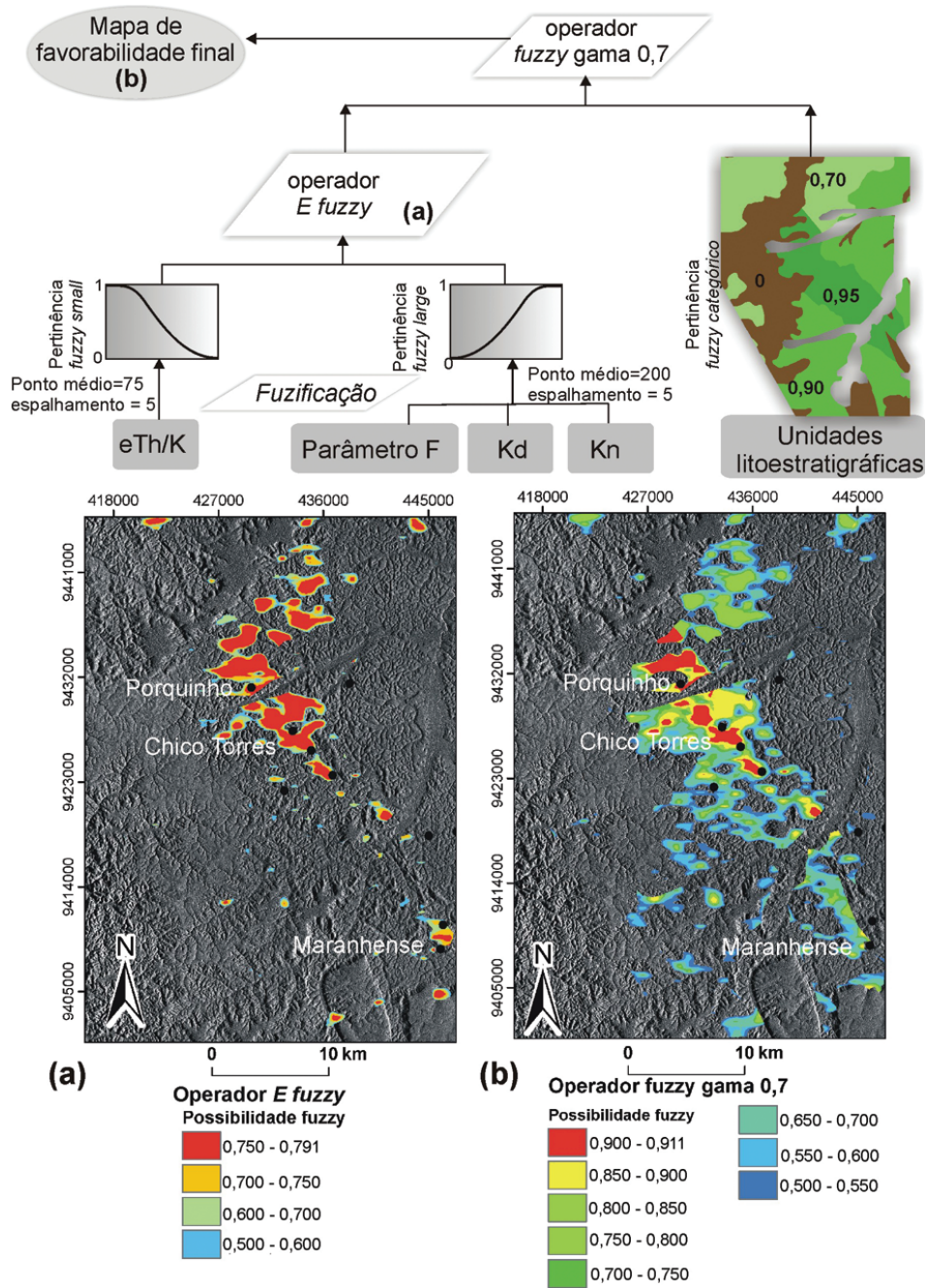
Figura 8 – Aplicação da lógica fuzzy na região da zona de cisalhamento Chico Torres. Os mapas de favorabilidade aurífera foram produzidos pelos seguintes operadores fuzzy : (a) E fuzzy ; (b) fuzzy gama (0,7).
