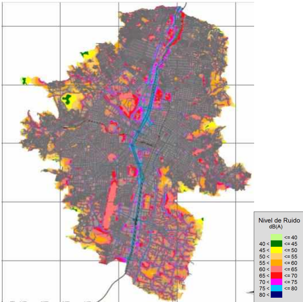
Mapa 2 - Ruído do trafego viário de Medellín: Dia.
