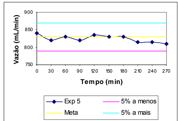
Figura B.4 – Vazão efluente ao longo do experimento 5
