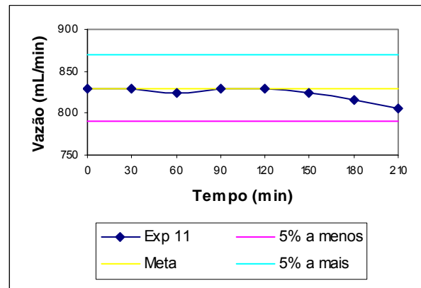
Figura B.10 – Vazão efluente ao longo do experimento 11
