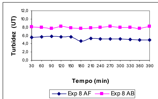
Figura C.8 – Turbidez da água bruta e da água filtrada ao longo do experimento 8
