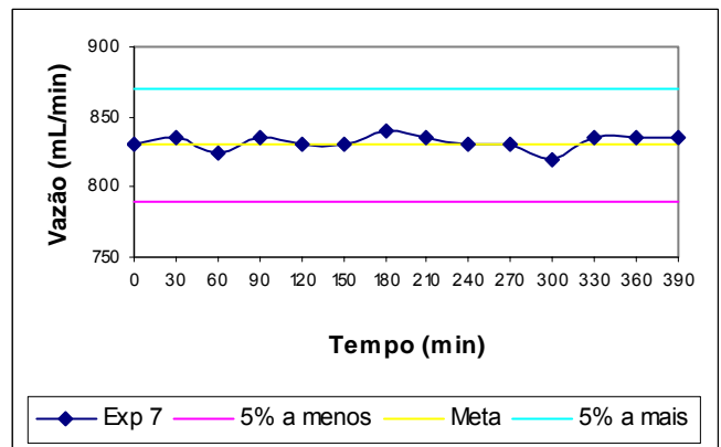
Figura B.6 – Vazão efluente ao longo do experimento 7
