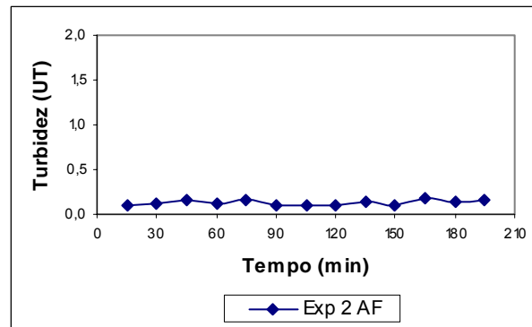
Figura C.2 – Turbidez da água filtrada ao longo do experimento 2
