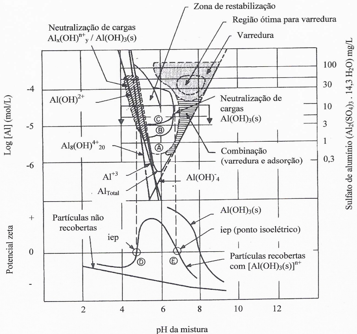
Figura 3.2 – Diagrama de coagulação com sulfato de alumínio e potencial zeta – Cleasby, 1990 (modificado)
