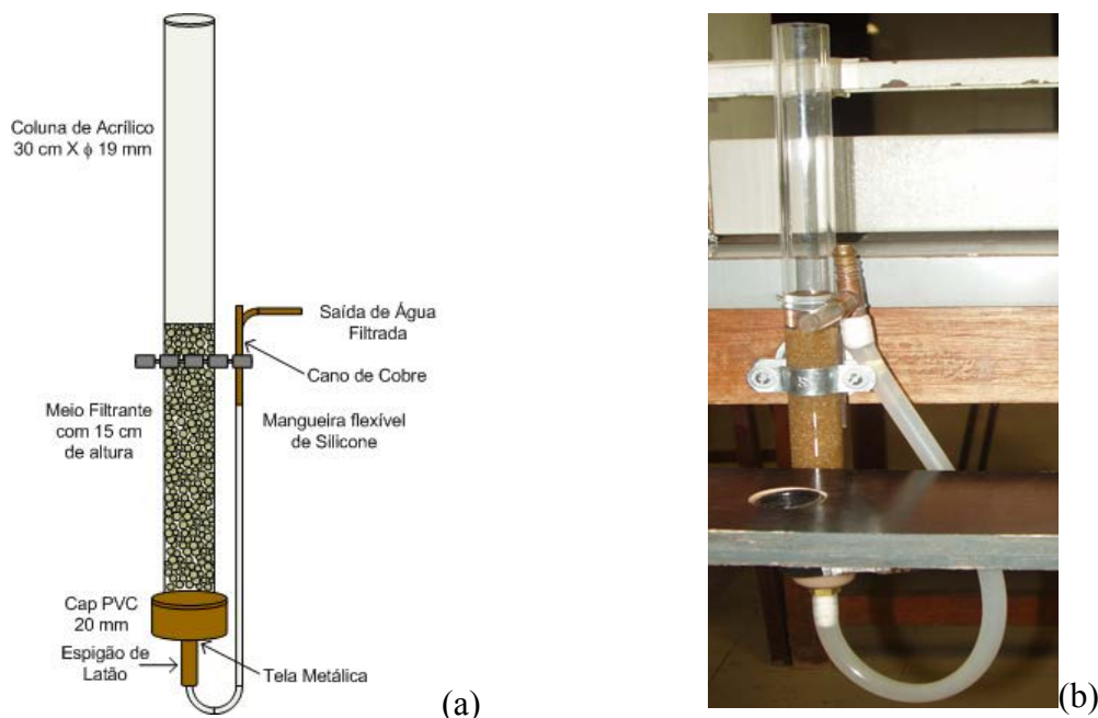
Figura 4.1 – Filtro de laboratório de areia (a) esquema; (b) foto
