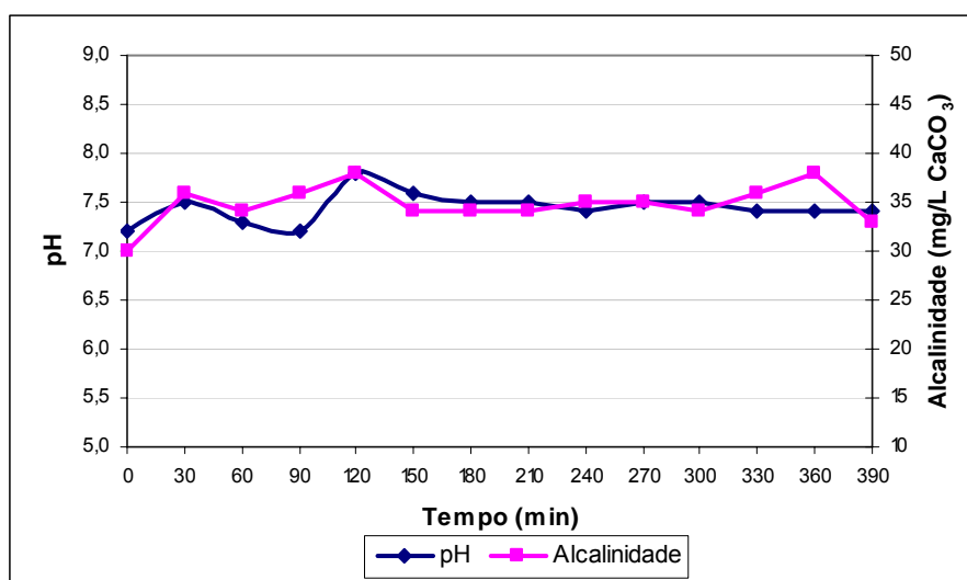
Figura 5.4 – Ensaios para a verificação da estabilidade do pH e da alcalinidade da água do córrego do Torto após alcalinização com bicarbonato de sódio – Fevereiro/2006
