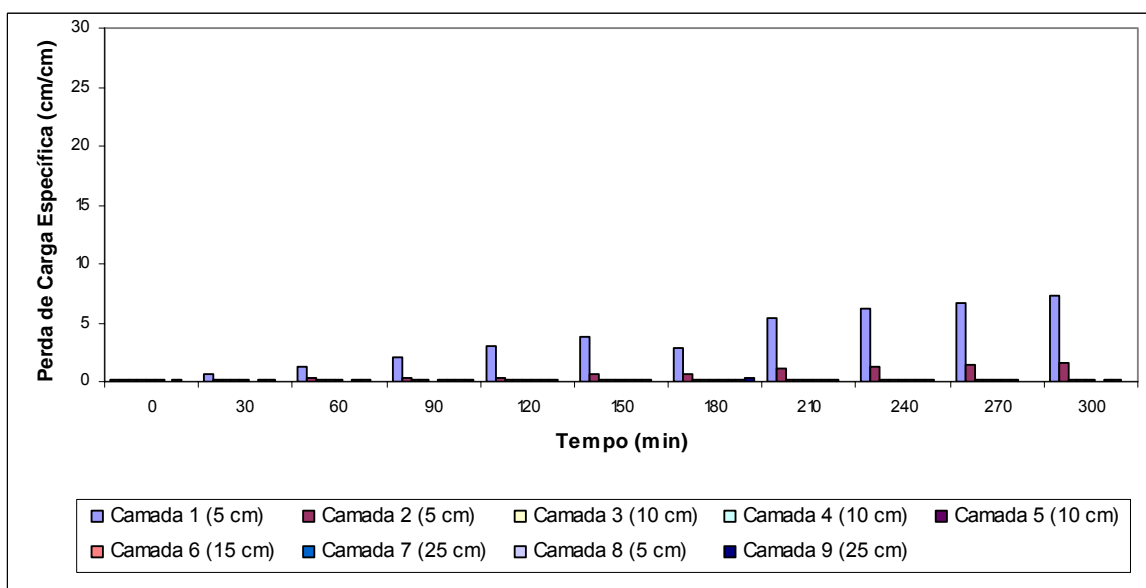
Figura D.10 – Taxa de crescimento das perdas de carga nas camadas do meio filtrante ao longo do experimento de filtração direta descendente – Experimento 10 Água do córrego do Torto em maio de 2006 – Taxa de filtração reduzida para 105 m 3 /m 2 dia
