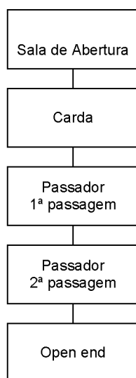
Figura A4.4 – Fluxograma do fio open end
