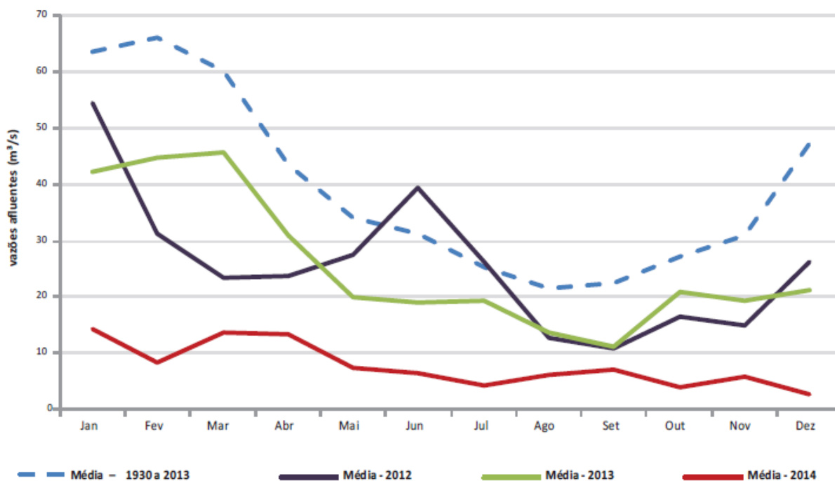
Figura 3 – Vazões mensais afluentes ao Reservatório Equivalente do Sistema Cantareira.
