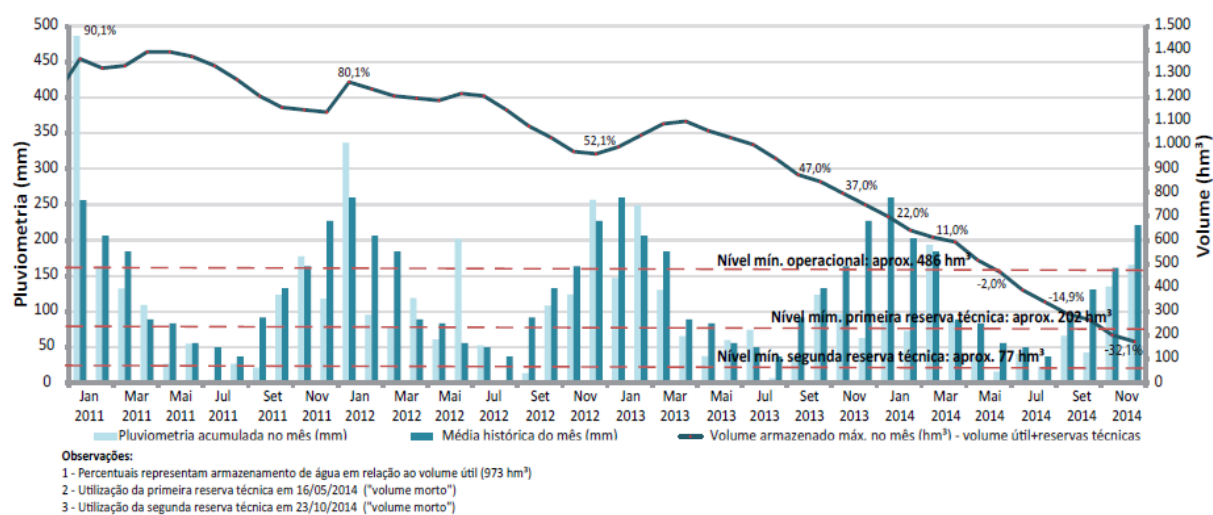
Figura 4 – Evolução do estoque de água no Sistema Cantareira de 2011 a 2014.
