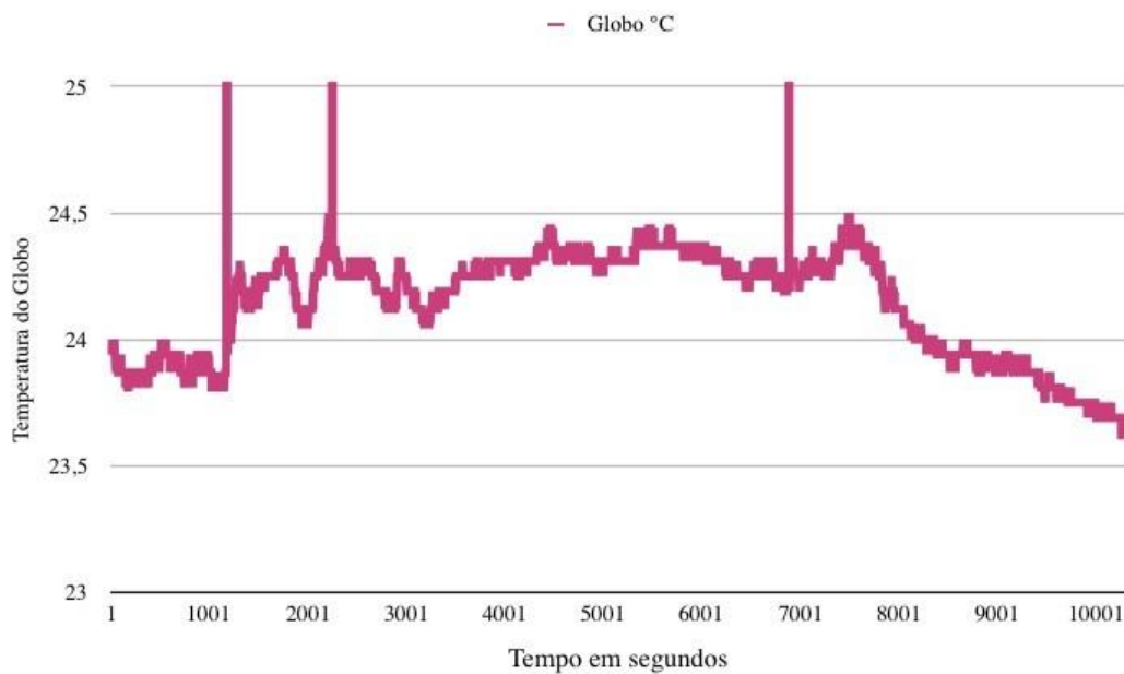
Figura 10 – Leitura da temperatura do globo negro
