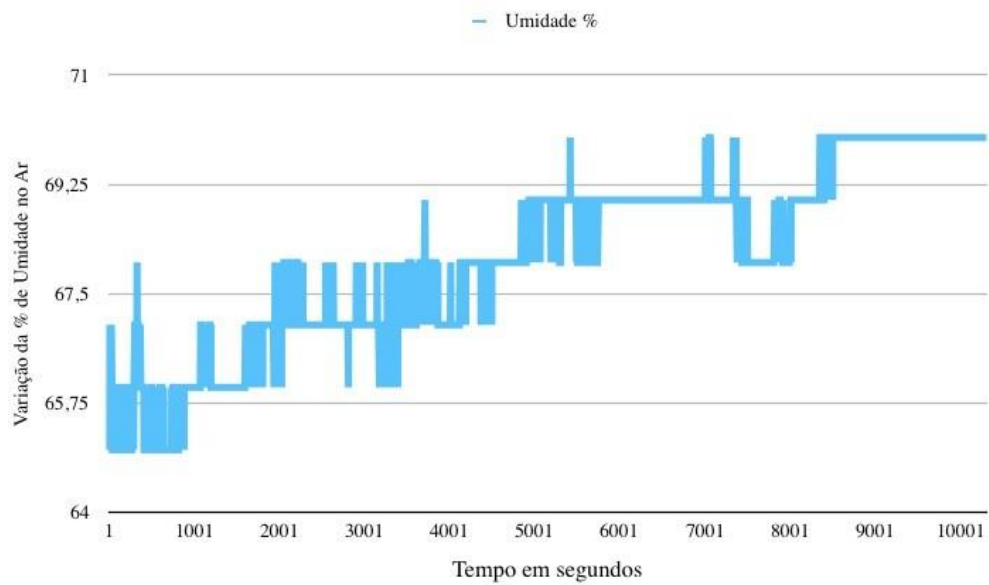
Figura 8 – Leitura da umidade relativa do ar com o sensor DHT11
