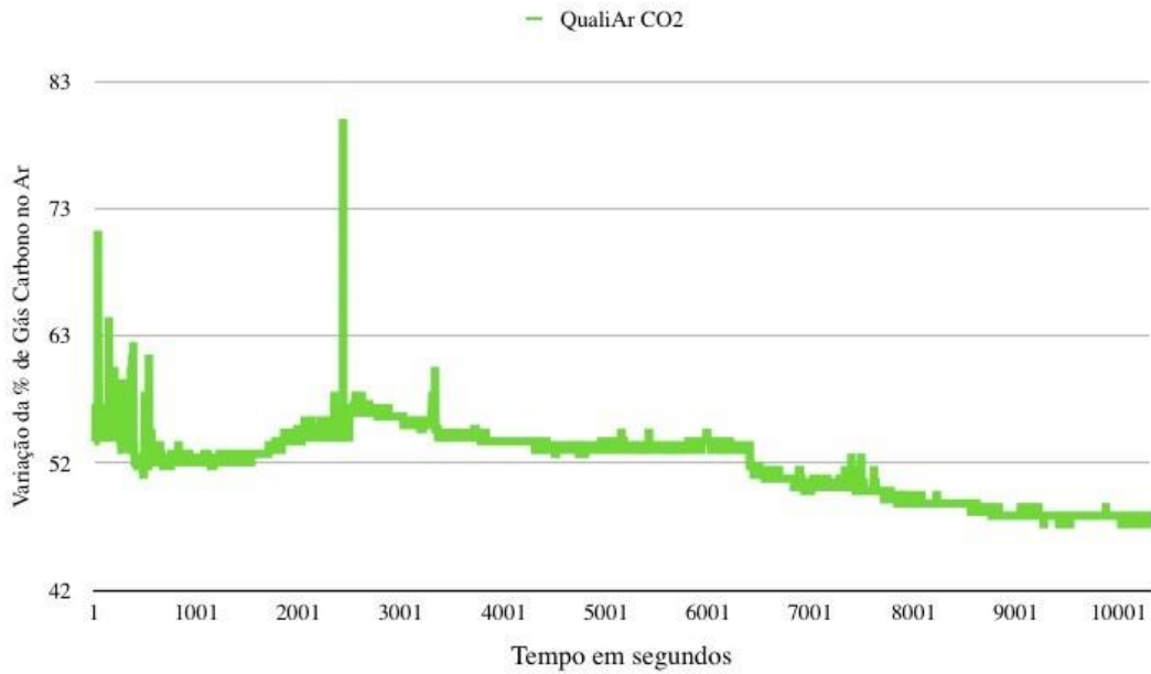
Figura 7 – Leitura do CO 2 coletados com o sensor MQ-135
