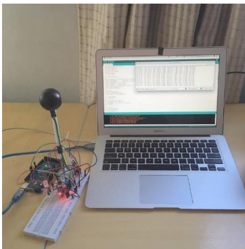
Figura 5 – Teste com o sensor de temperatura de globo.
