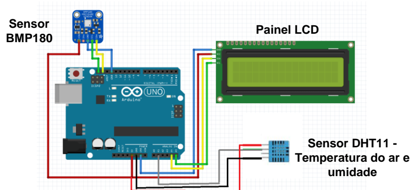
Figura 1 – Esquema de montagem da placa utilizada no sistema da mochila bioclimática.
