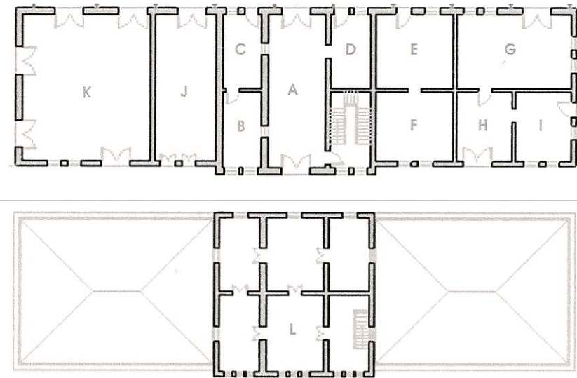
Figura 30 – Planta da Estação de São João Del Rei.
