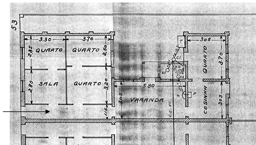
Figura 95 – Planta baixa de uma unidade do Tipo 2
